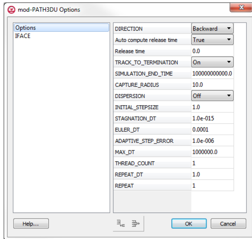
Figure 3 mod-PATH3DU Options dialog.
